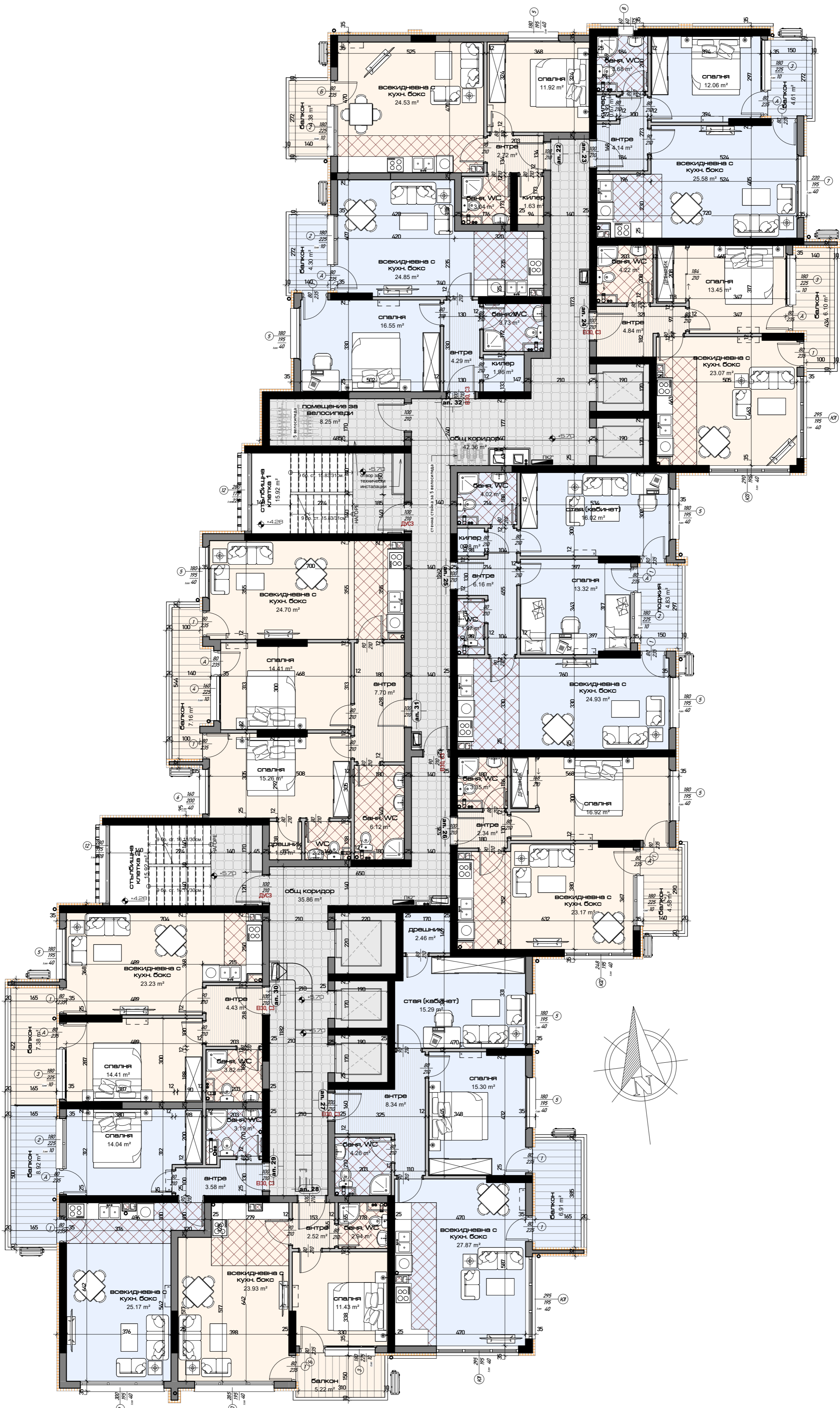
9 РАЗПРЕДЕЛЕНИЕ ЕТАЖ 4 (кт. +5.70м.)
