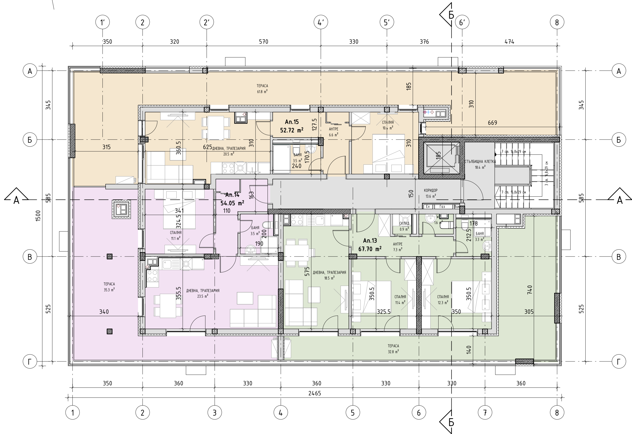
РАЗПРЕДЕЛЕНИЕ КОТА +9.15 М 1:100
